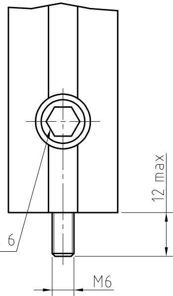
DETAIL X M 1:1
