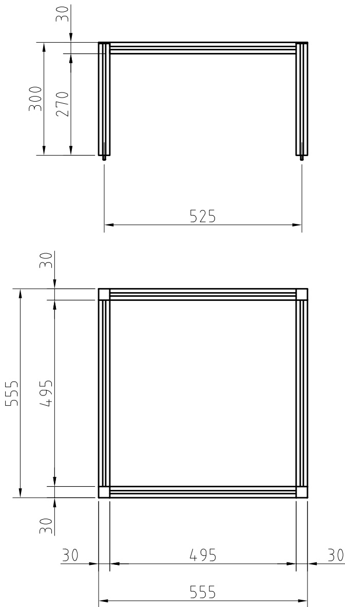
DETAIL X M 1:1
