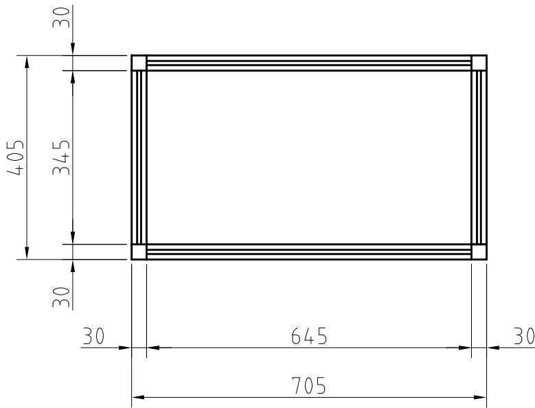
DETAIL X M 1:1
