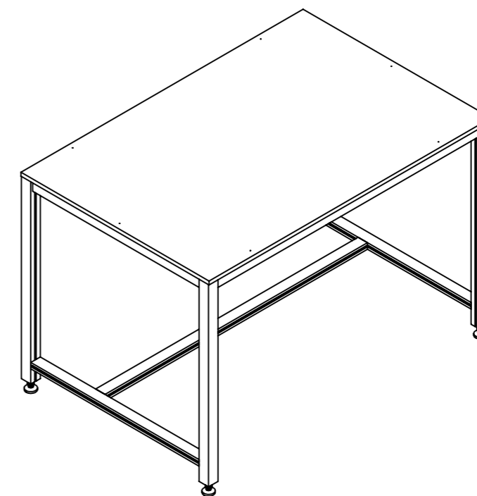
Stůl pracovní SPR4NST-1x1,5x1-A1xLDT
